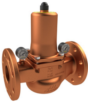
Flanschen-Druckminderer, Figur 711 00
