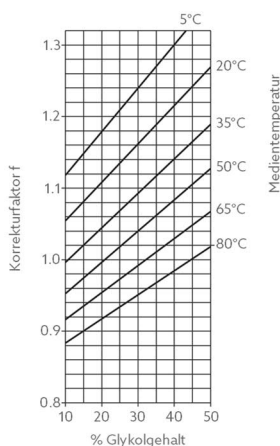
Korrekturfaktor f für Ethylen Glykol
